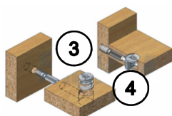
Эксцентриковая стяжка
