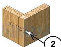
Евровинт 7 x 50
